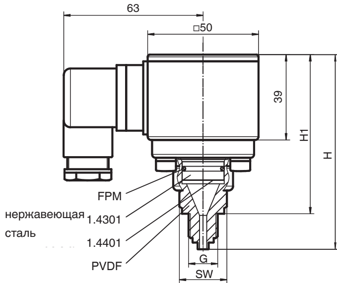
Пример конструкции датчика, код материала датчика A0
